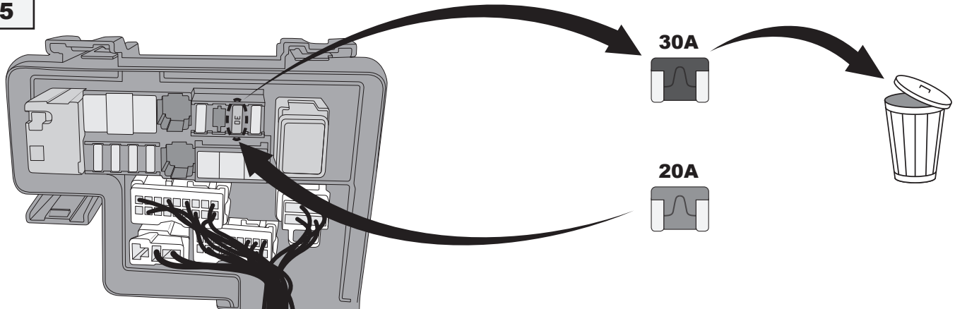
Sicherung 20A → Sicherungskasten fuse 20A → fusebox
