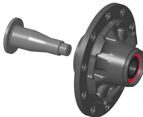
Obrázek 2: Náboj kola s FAG SmartSET pro nápravy BPW
