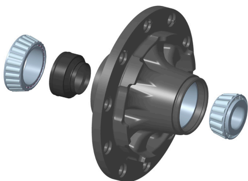
Obrázek 1: Kartuše s mazivem (černá) náboje kola pro nápravy BPW
