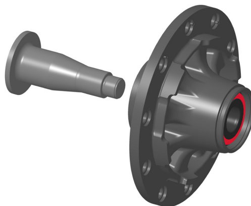
2. ábra: Kerékagy FAG SmartSET-tel a BPW-tengelyekhez
