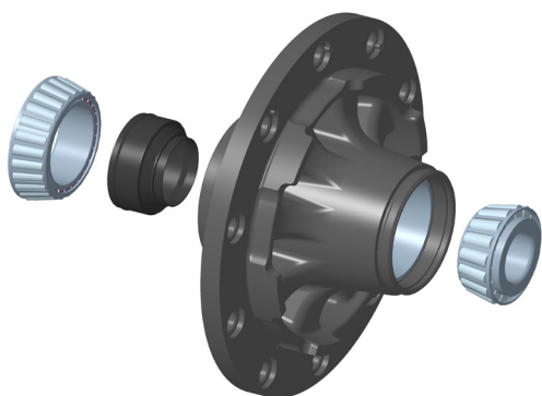
1. ábra: Egy BPW-tengely kerékagyának zsírpatronja (fekete)
