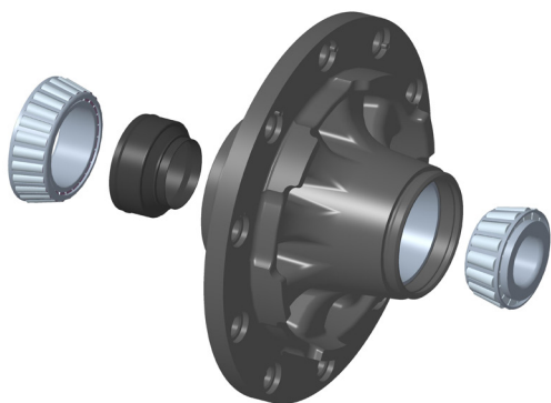
Fig. 1: Cartucho de massa lubrificante (preto) de um cubo de roda para eixos BPW
