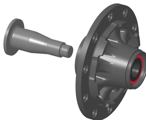
Fig. 2: Cubo de roda com FAG SmartSET para eixos BPW
