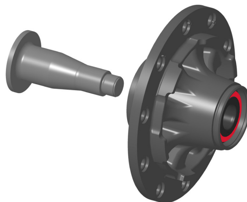
Figura 2: Butuc de roată cu FAG SmartSet pentru axe BPW
