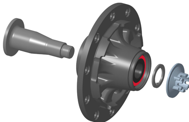
Bild 2: Radnabe mit geänderter Anlaufscheibe und Achsmutter mit großem Bund
