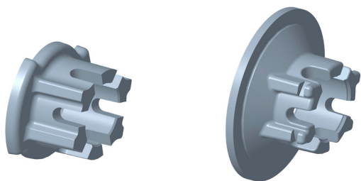
Bild 1: Achsmutter mit kleinem (links) und großem (rechts) Bund
