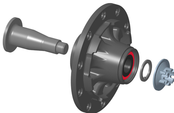
Afbeelding 2: Wielnaaf met gewijzigde aanloopschijf en asmoer met grote kraag
