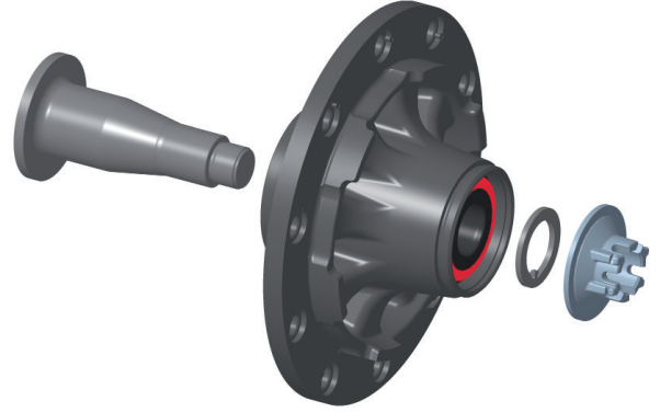
Şekil 2: Değiştirilmiş baskı pulu olan porya ve daha geniş yakalı aks somunu
