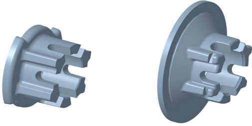
Şekil 1: Dar (sol) ve geniş (sağ) yakalı aks somunu
