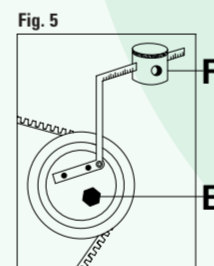
FIGURA 5 Allentare il bullone di bloccaggio E, inserire l'apposito attrezzo di tensionamento con il relativo peso F-100 mm (per motori 16V); 140 mm (per motori 8V). Verificare che il braccio dell'attrezzo rimanga in posizione orizzontale; serrare, quindi, il bullone di bloccaggio E.
