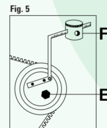
FIGURA 5 Aflojar el tornillo de fijación E. Insertar la herramienta específica para tensado de correas con su peso relativo. (F:100 mm para motores 16V; (F):140 mm para motores V6). Verificar que el brazo de la herramienta permanezca en posición horizontal. Por último, apriete el tornillo de fijación E.
