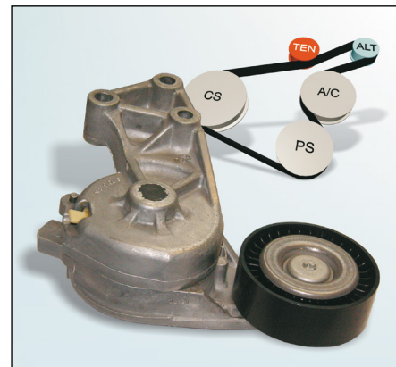
Slika 2: Jedinica za natezanje remena Kat. Br. 534 0132 30 namijenjena za motor 1,9 TDI s prikazom pravilnog kretanja remena
