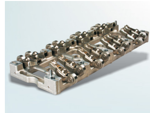
Kuva 1: Keinuviivun laakerin teline 423 0061 10
