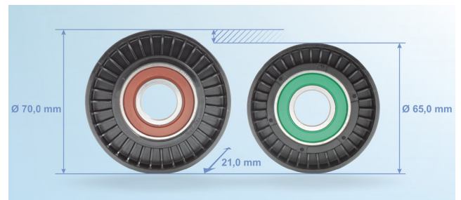
Kuva 2: Ohjainpyörä 532 0404 30 ottomoottorilla varustettuihin autoihin (vasemmalla) ja ohjainpyörä 532 0406 30 dieselmoottorilla varustettuihin autoihin (oikealla)
