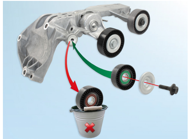
Kuva 1: Hihnankiristin 534 0243 10
