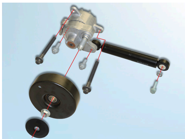
1. ábra: 533 0116 10 – INA javítókészlet a segédberendezések hajtásához a rögzítőcsavarokkal együtt
