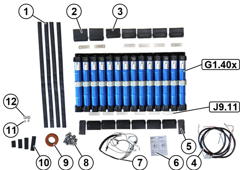
Abbildung 1 HV- Batterie Reparatursatz Kit - Lieferumfang
