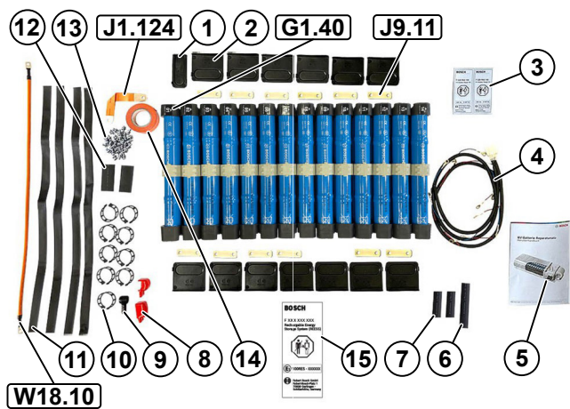
Afbeelding 1 HV-accureparatieset - leveringsomvang
