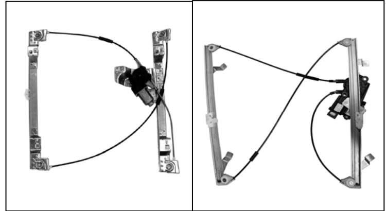
Elevavinas original – lève-vitre original / oem window regulator – levandador de vidro original Nuestro elevavinas – notre lève-vitre / our window regulator – nosso levandador de vidro
