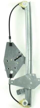
Nuestro Elevallunas / Our window regulator / Notre lève-vitre / Nosso elevador de vidro
