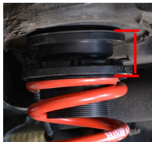
Abb. 5: Einstellmaß HA
