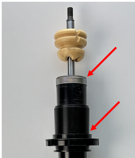
Abb. 2: Höhenverstellung und Abdeckkappe mont.
