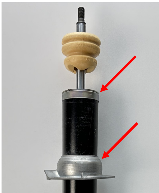
Abb. 1: Abdeckkappe und Federteller demontieren
