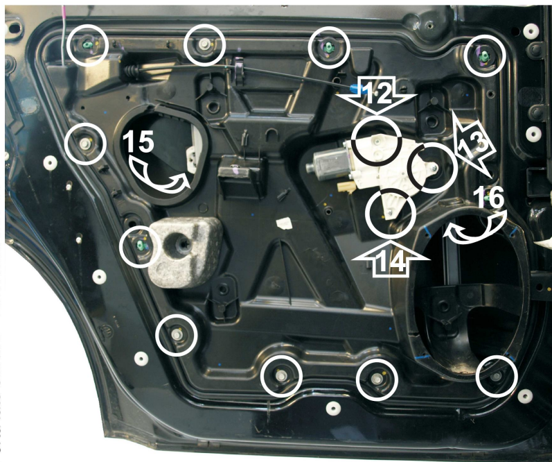
Porta lato sinistro - Left hand side door
