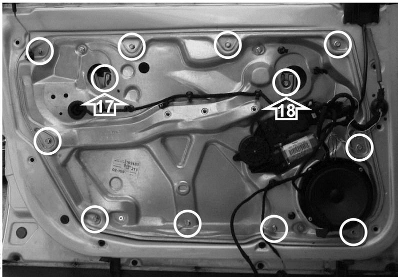
Porta lato sinistro - Left hand side door
