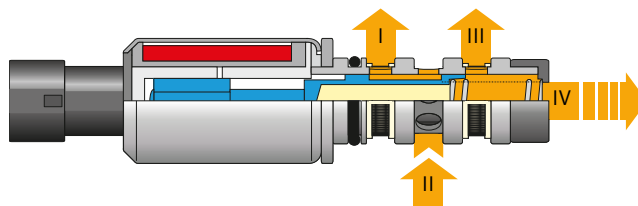
Ranhura do anel I - III e retorno IV na válvula de comando
