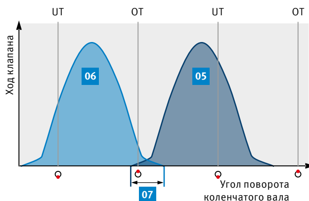
Перекрытие клапанов
