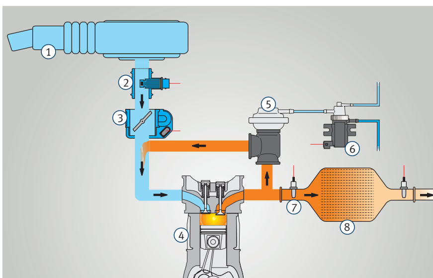
Princip recirkulacije izduvnih gasova (pneumatski)
