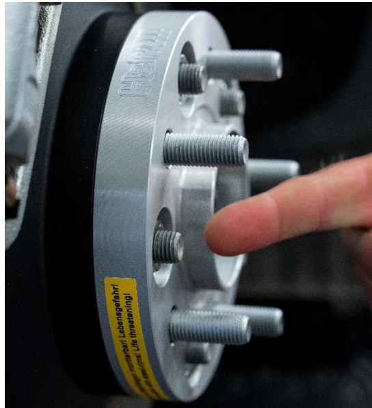
Überstand der originalen Stehbolzen nach Verbau der Spurverbreiterungen Overhang of the original studs after installation of the wheel spacers
