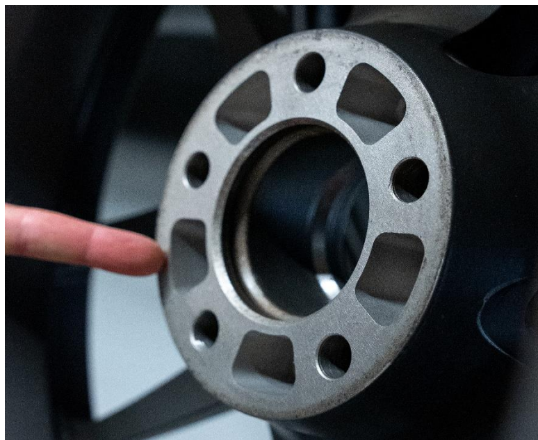
Gießtaschen in den Rädern / Cast holes of the wheels
