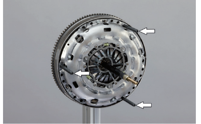
Resim 2: Taşıyıcı aparatı sabitlemek için saplama cıvataları
