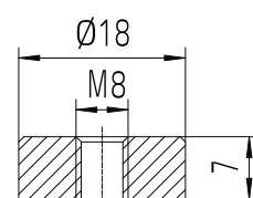
Polausführung F-M8
