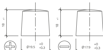
Polausführung 1
